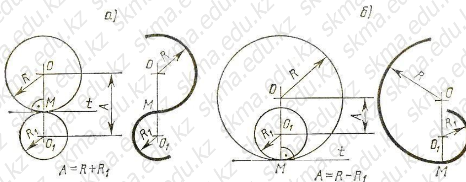
РИС. 15 ВНЕШНЕЕ И ВНУТРЕННЕЕ КАСАНИЕ ДВУХ ДУГ
