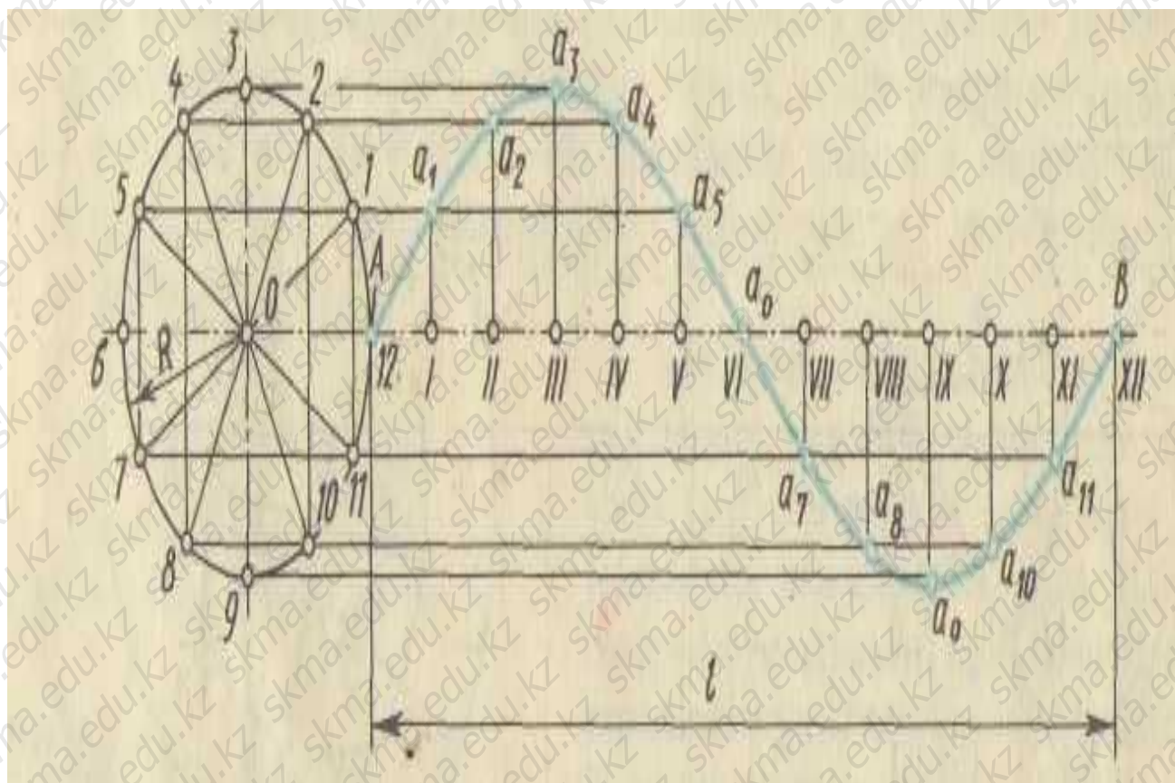
Рис. 20. Построение синусоиды.
